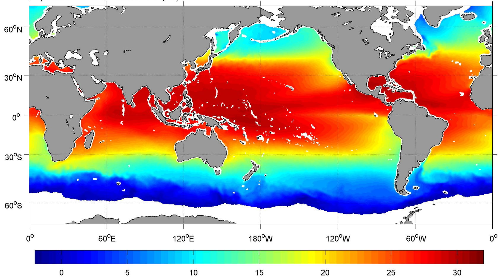
September SCOW AMSR SST (°C)
