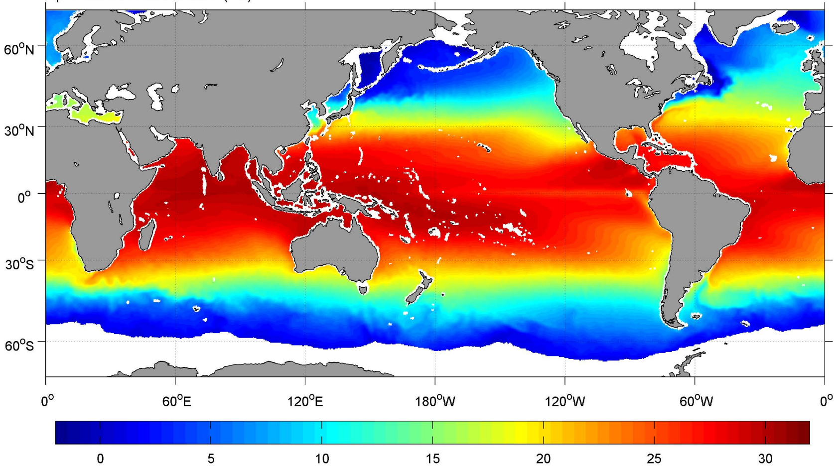
April SCOW AMSR SST (°C)
